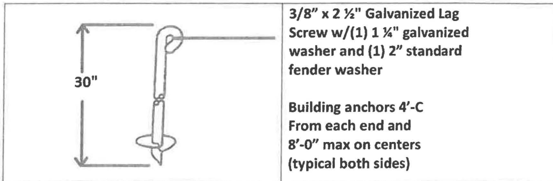
Building Anchor Detail (N.T.S.)
